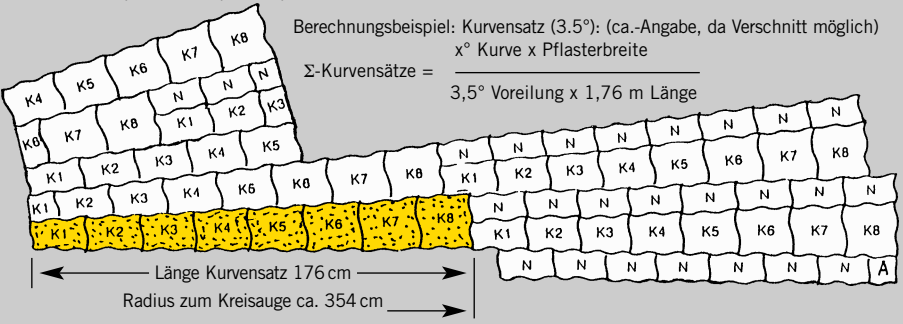
PW im Läufer-Verband – gefast u. scharfkantig
